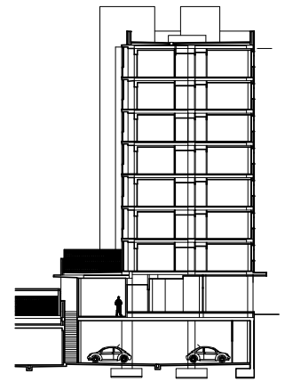
SECCIÓN
