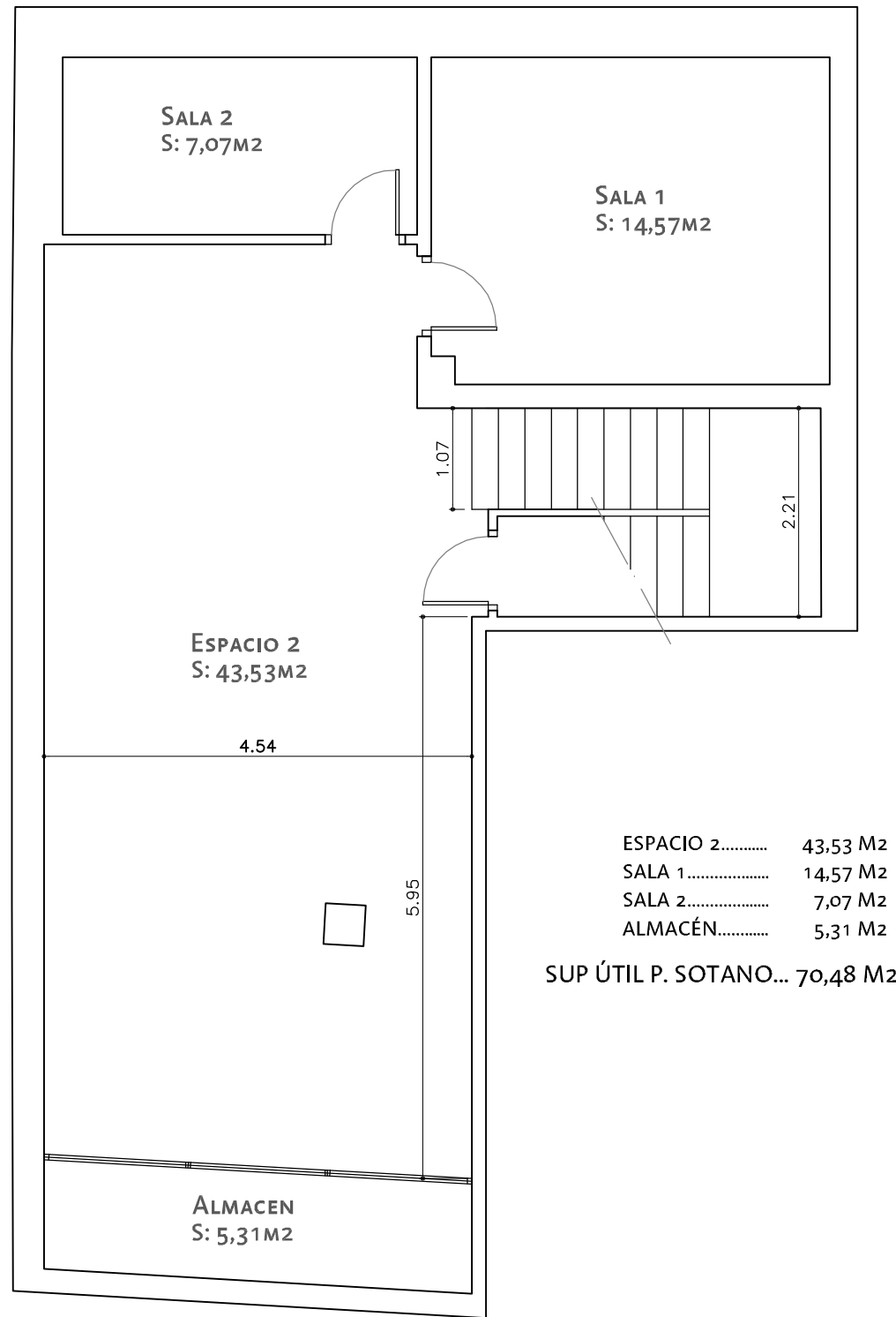
PLANTA SOTANO
